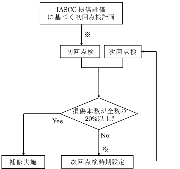
※ 予防保全を選択することも可能 図 2.2.2-1 点検・評価フロー
